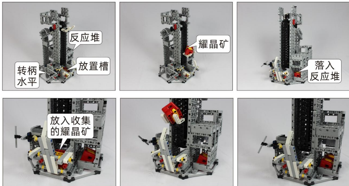
图 6 反应堆运行的初始及完成状态
